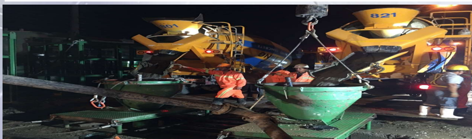
งานเจาะเสาเข็ม Barrette Pile 1.00x3.80 m. MLP08-11C No.2
