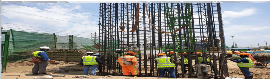
งานเจาะเสาเข็ม Barrette Pile 1.00x3.80 m. MLP06-15 No.2
